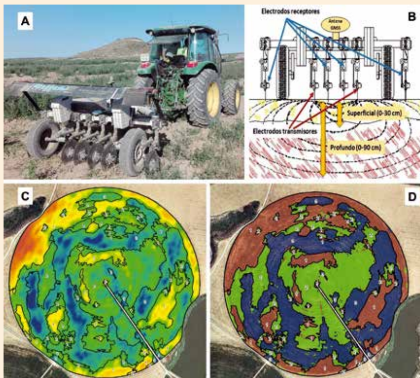
A) Medidor de CEa Veris 3100 que permite conocer la conductividad eléctrica aparente del suelo a dos profundidades, superficial (de 0 – 30 cm) y profunda (de 0 90 cm) mediante un sistema de electrodos que inyectan corriente continua y otros receptores que miden la conducción de dicha corriente a través del suelo (B). C) Mapa de la CEa en un pivó de 30 ha que muestra la variabilidad de esta propiedad que se puede relacionar con el potencial productivo del suelo. D) Mapa de zonas derivado del mapa de la CEa con la definición de zonas de manejo para aplicar diferentes dosis de siembra y fertilización de maíz.
